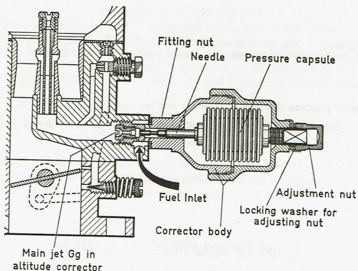
Fig. 41 SOLEX Altitude Corrector
